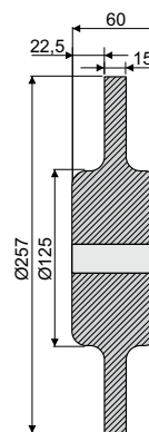
SECCIÓN A-A
