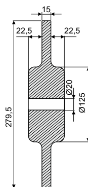
SECCIÓN A-A ESCALA 1 : 1
