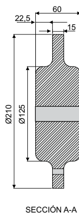
SECCIÓN A-A
