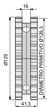
SECCIÓN A-A
